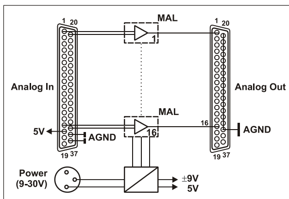
Funktionsschaltbild
