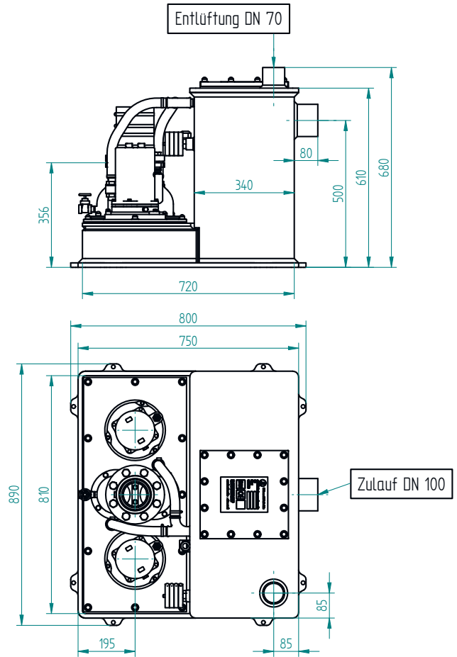
Baumaße HEBESTAR 320 Duplex
