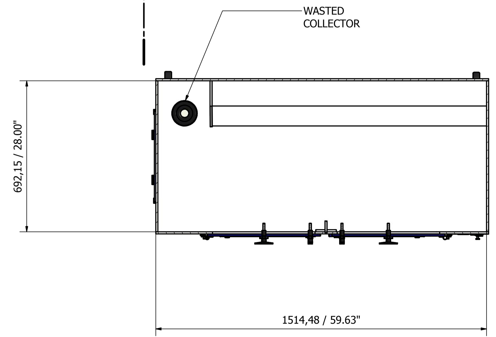
B-B ( 1 : 10 )
