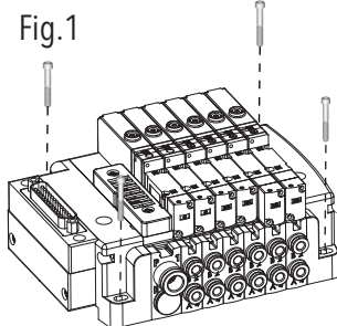
With through screws. Avec vis traversantes. Con viti passanti.
