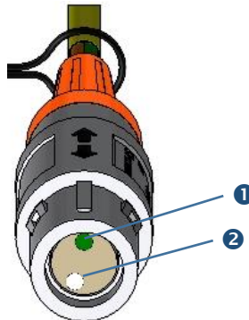
Abb. 2: Belegung des Anschlusssteckers (Ansicht auf Stiftseite)
