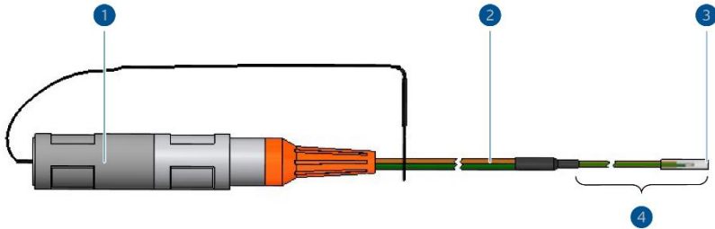
Abb. 1: Aufbau der HV Temperatursensor R58-HV-1Ka-xxx
