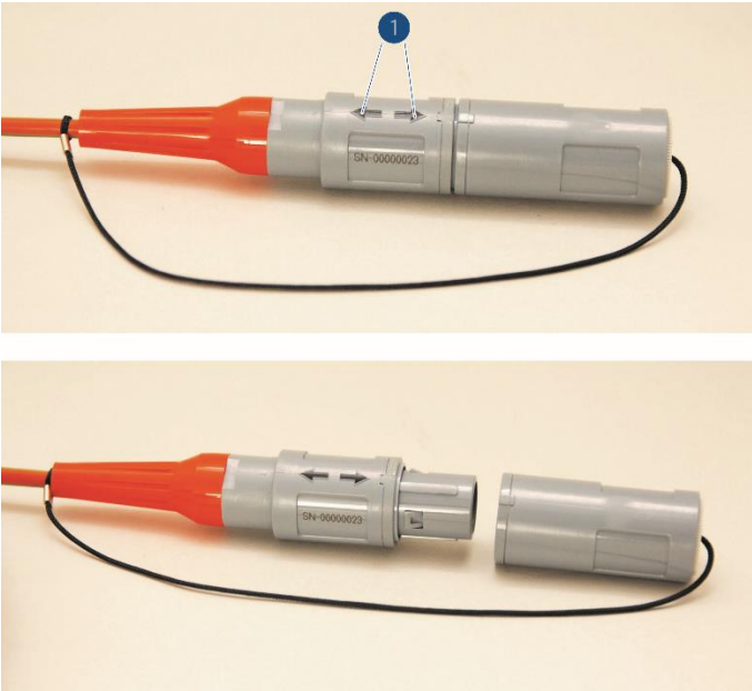
Abb. 3: Betätigen des Verriegelungsring beim Abnehmen der Abdeckkappe
