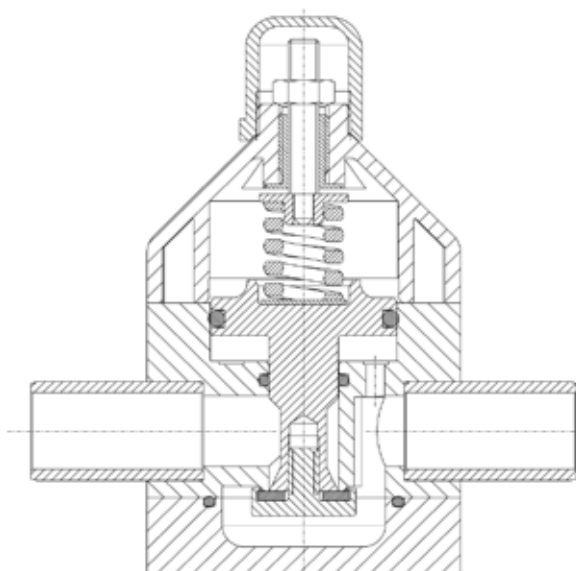
Schnittbild
