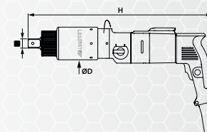
Gerade Ausführung
