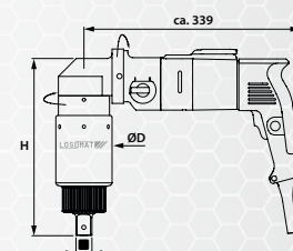
Abgewinkelte Ausführung
