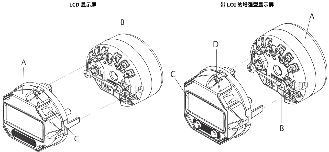
图 11: 显示单元
